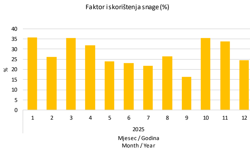
Slika 10 Mjesečni faktor iskorištenja snage svih vjetroelektrana
