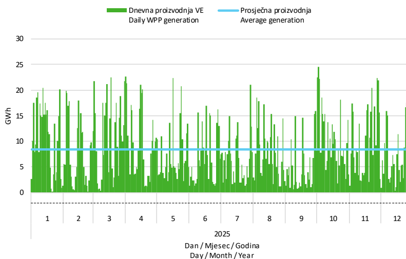
Slika 6 Dnevna proizvodnja svih vjetroelektrana
