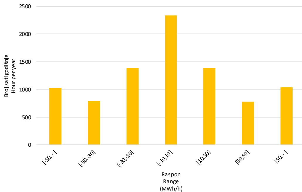
Slika 14 Statistička raspodjela satnih promjena proizvodnje VE
