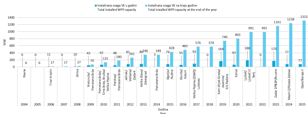
Slika 2 Vremenska dinamika izgradnje VE u Hrvatskoj
