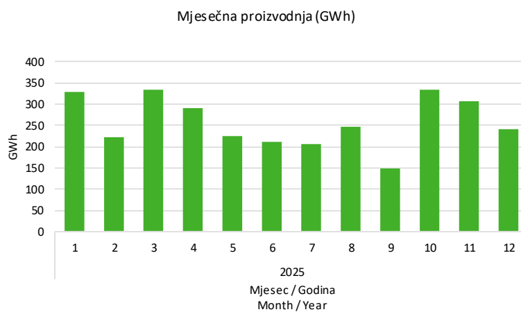
Slika 9 Mjesečna proizvodnja svih vjetroelektrana
